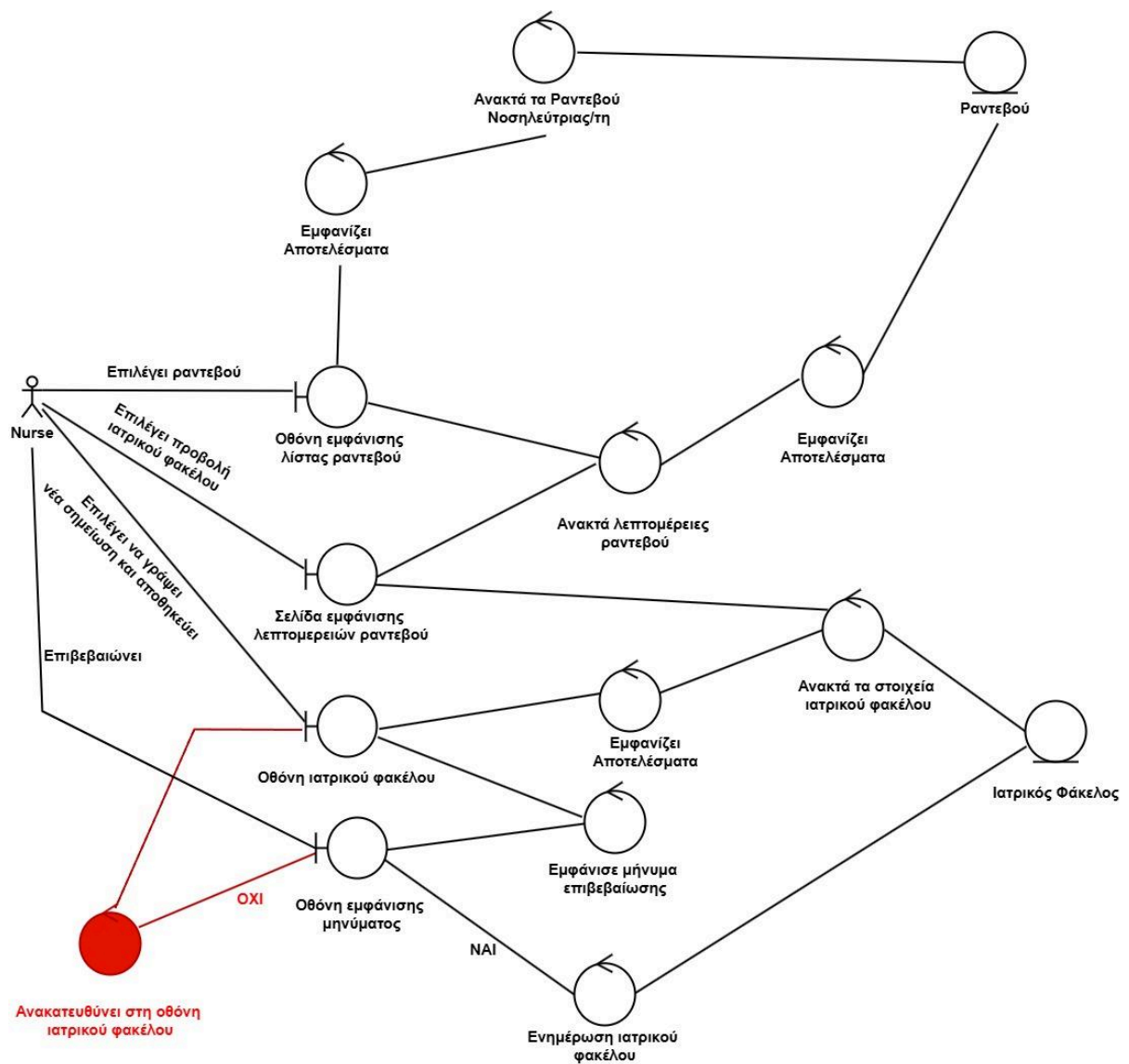
Robustness Diagram B: Πρόσβαση και ενημέρωση ιατρικού φακέλου
