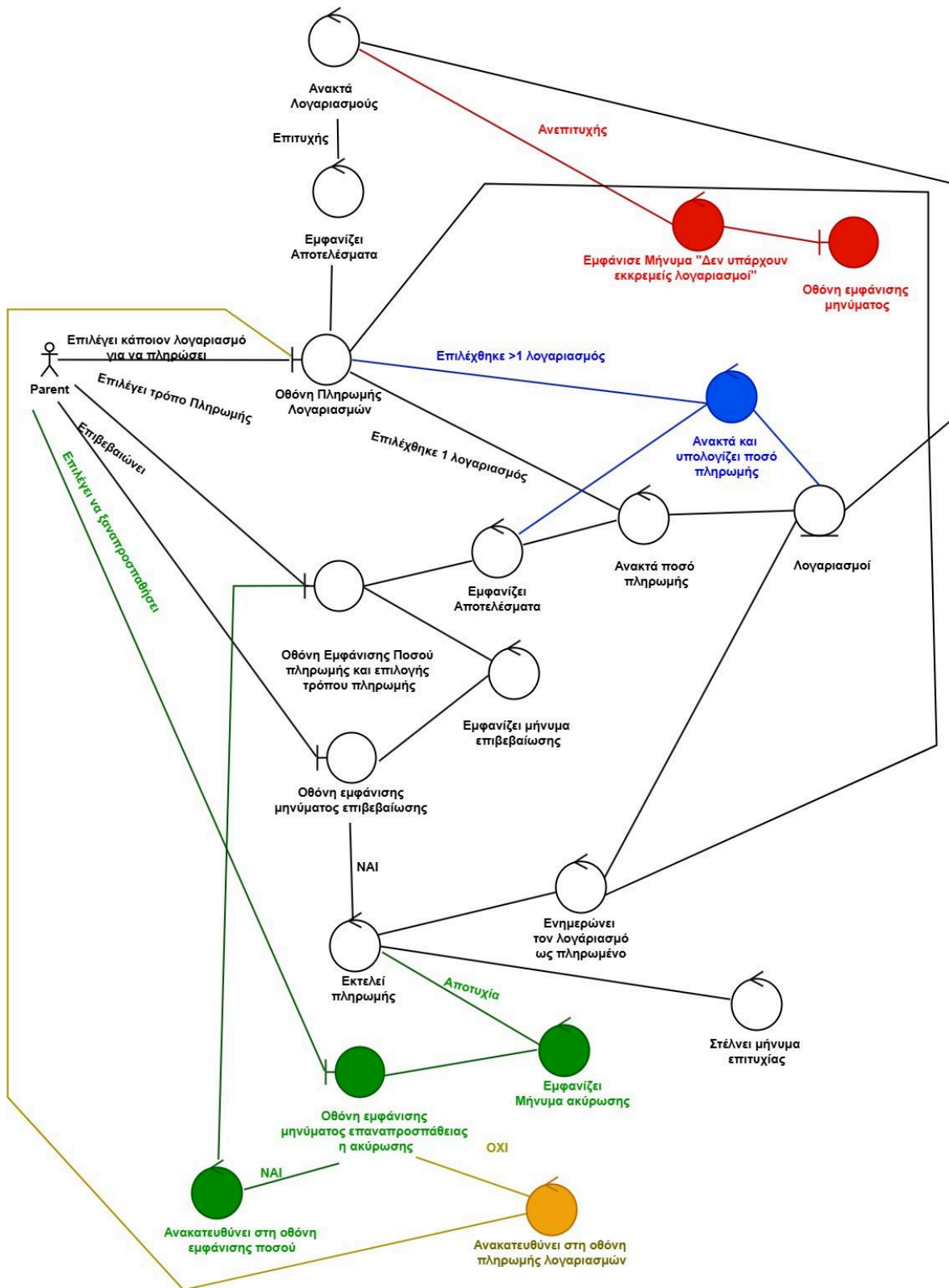
Robustness Diagram 2: Πληρωμές λογαριασμών
