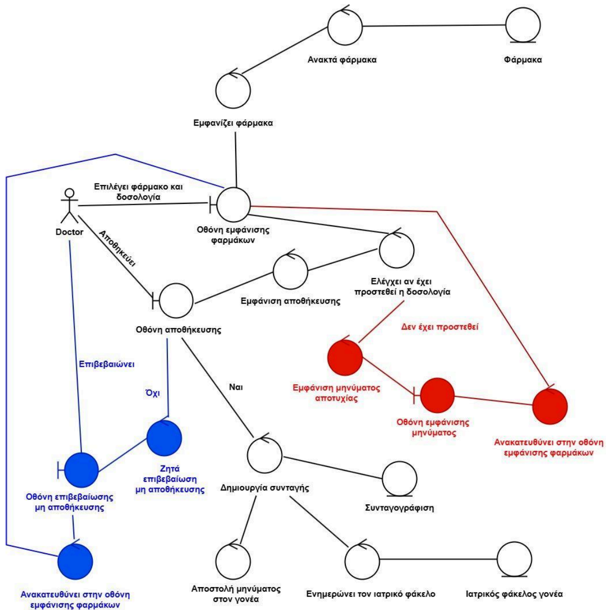
Robustness Diagram 9: Συνταγογράφηση
