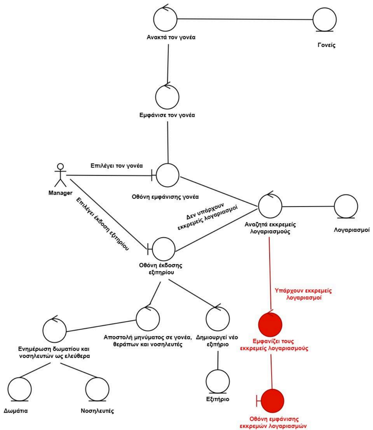
Robustness Diagram 6: Εκδοση εξιτηρίου
