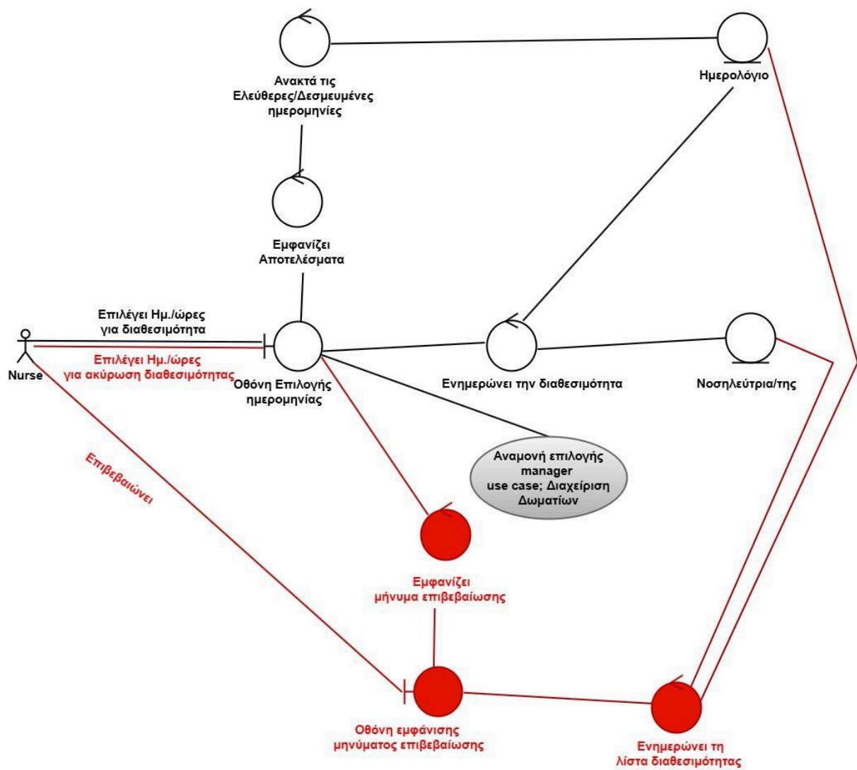
Robustness Diagram A: Δήλωση διαθεσιμότητας
