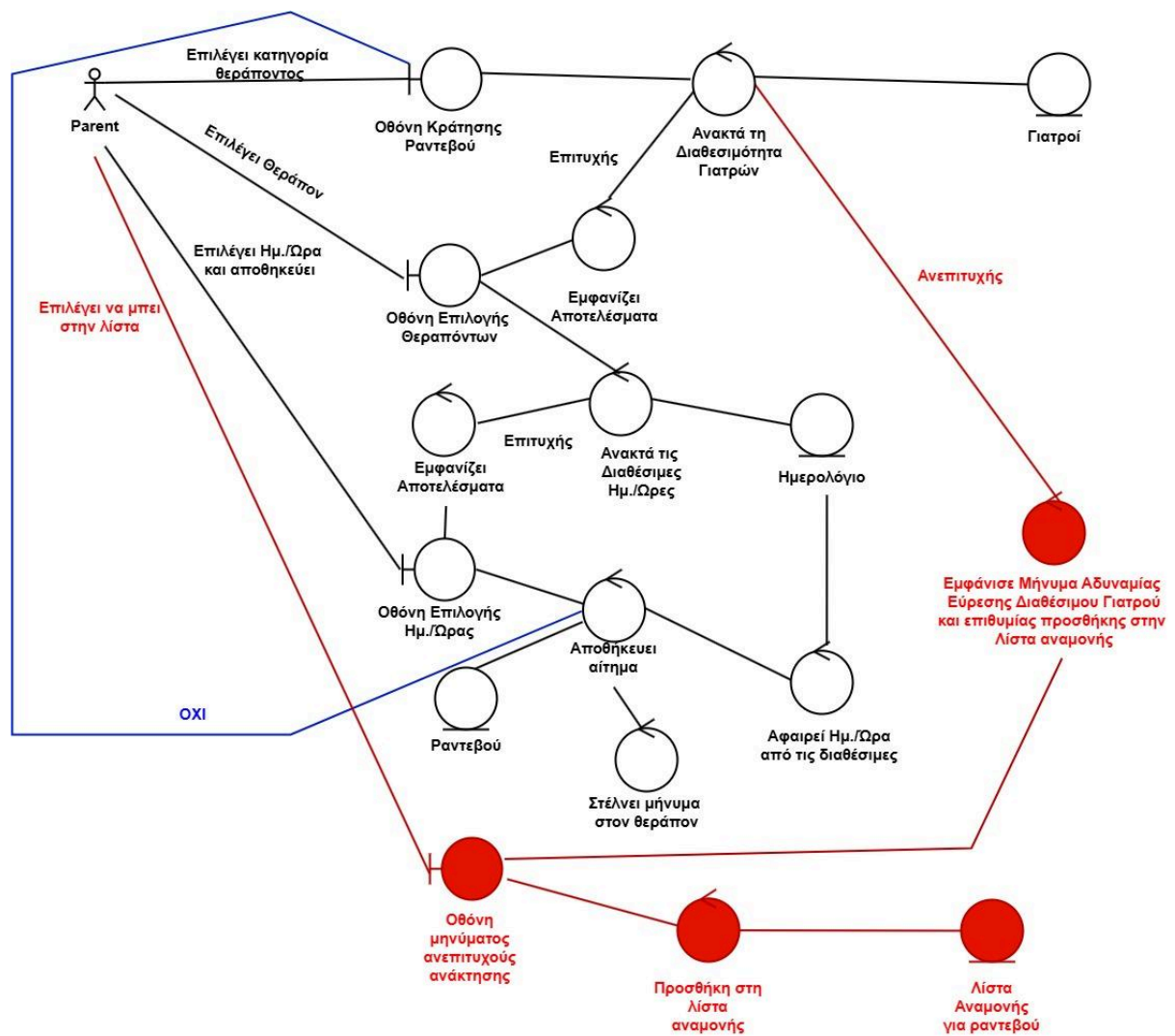
Robustness Diagram 1: Προγραμματισμός ραντεβού
