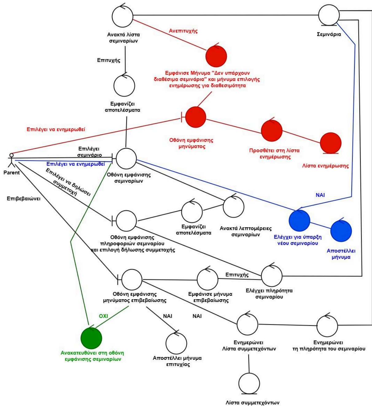
Robustness Diagram 3: Συμμετοχή σε σεμινάρια
