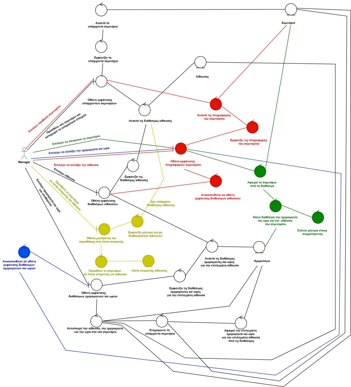
Robustness Diagram 5: Διαχείριση σεμιναρίων
